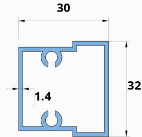
GRILL MIDDLE 30 Section Number - SA 54 Weight ( KG/M ) - 0.509
