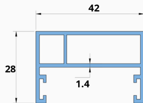
GRILL FRAME 42 Section Number - SA 53 Weight ( KG/M ) - 0.574
