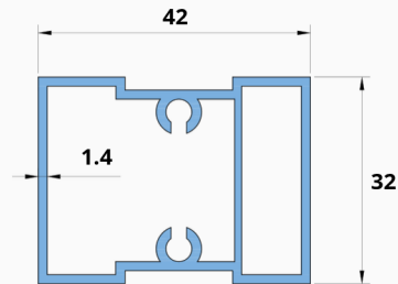
GRILL MIDDLE 42 Section Number - SA 40 Weight ( KG/M ) - 0.708
